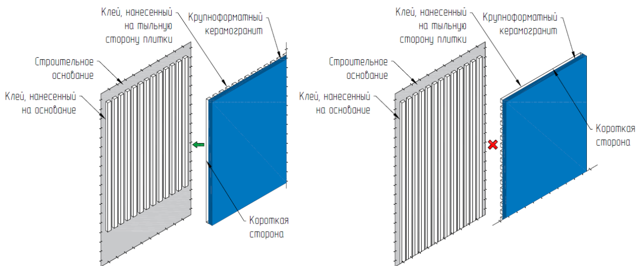
Рис. 22. Клей следует наносить в одном направлении на основание и на плитку
