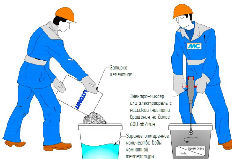
Рис. 30. Приготовление состава
