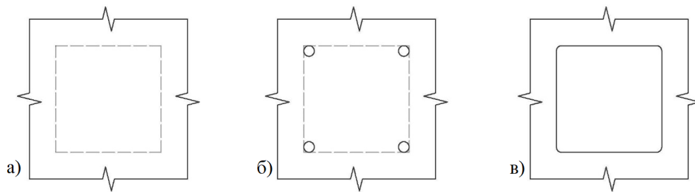
Рис. 25. Резка прямоугольных отверстий
