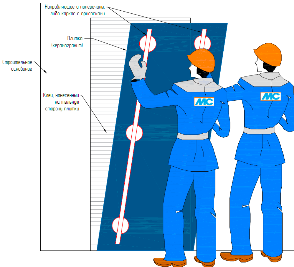
Рис. 26. Монтаж крупноформатного керамогранита
